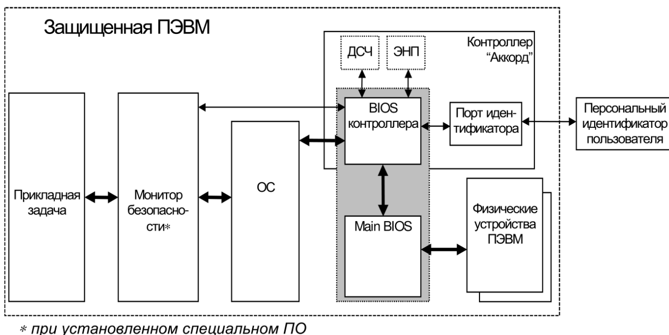
Рисунок 1 - Построение системы защиты информации от НСД с использованием комплекса «Аккорд-АМДЗ»
